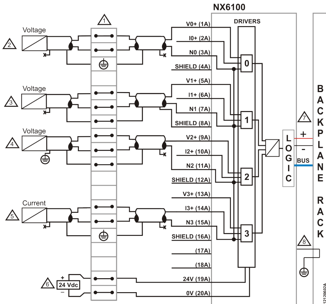
Figura 3: Diagrama Elétrico
