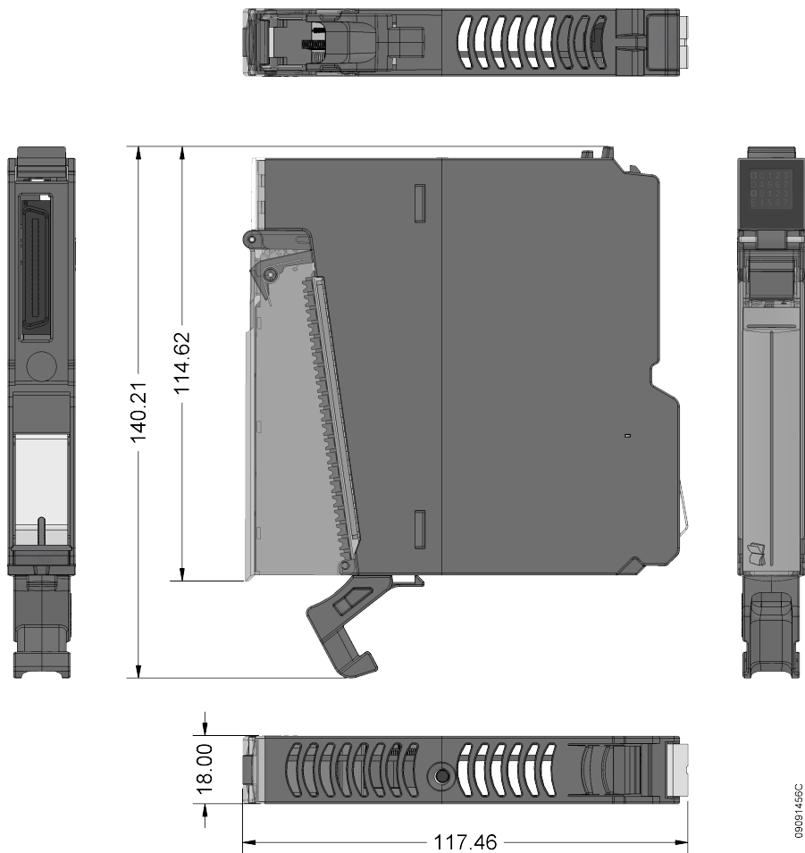
Figura 1: Dimensões Físicas
