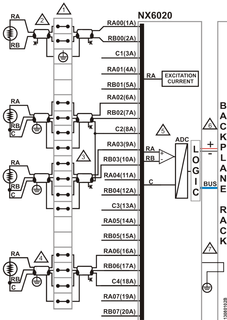
Figura 3: Diagrama Elétrico
