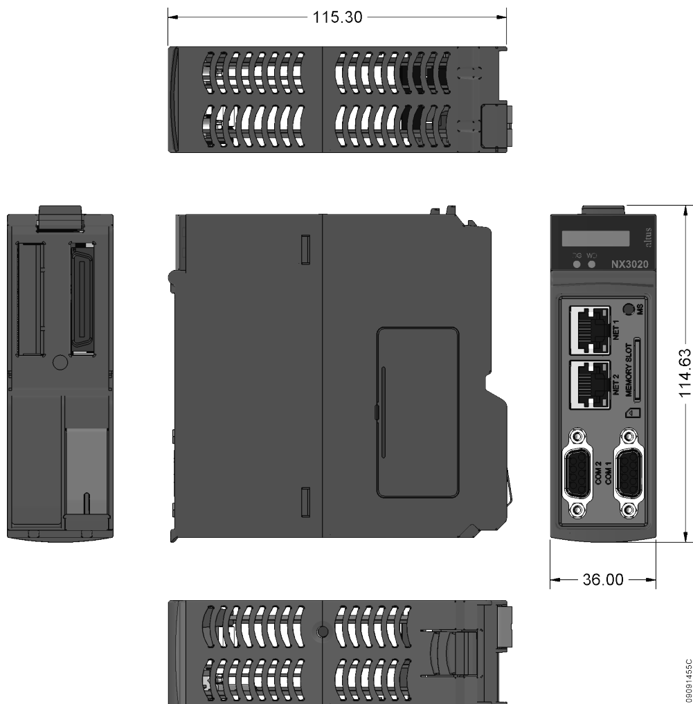
Figura 1: Dimensões Físicas
