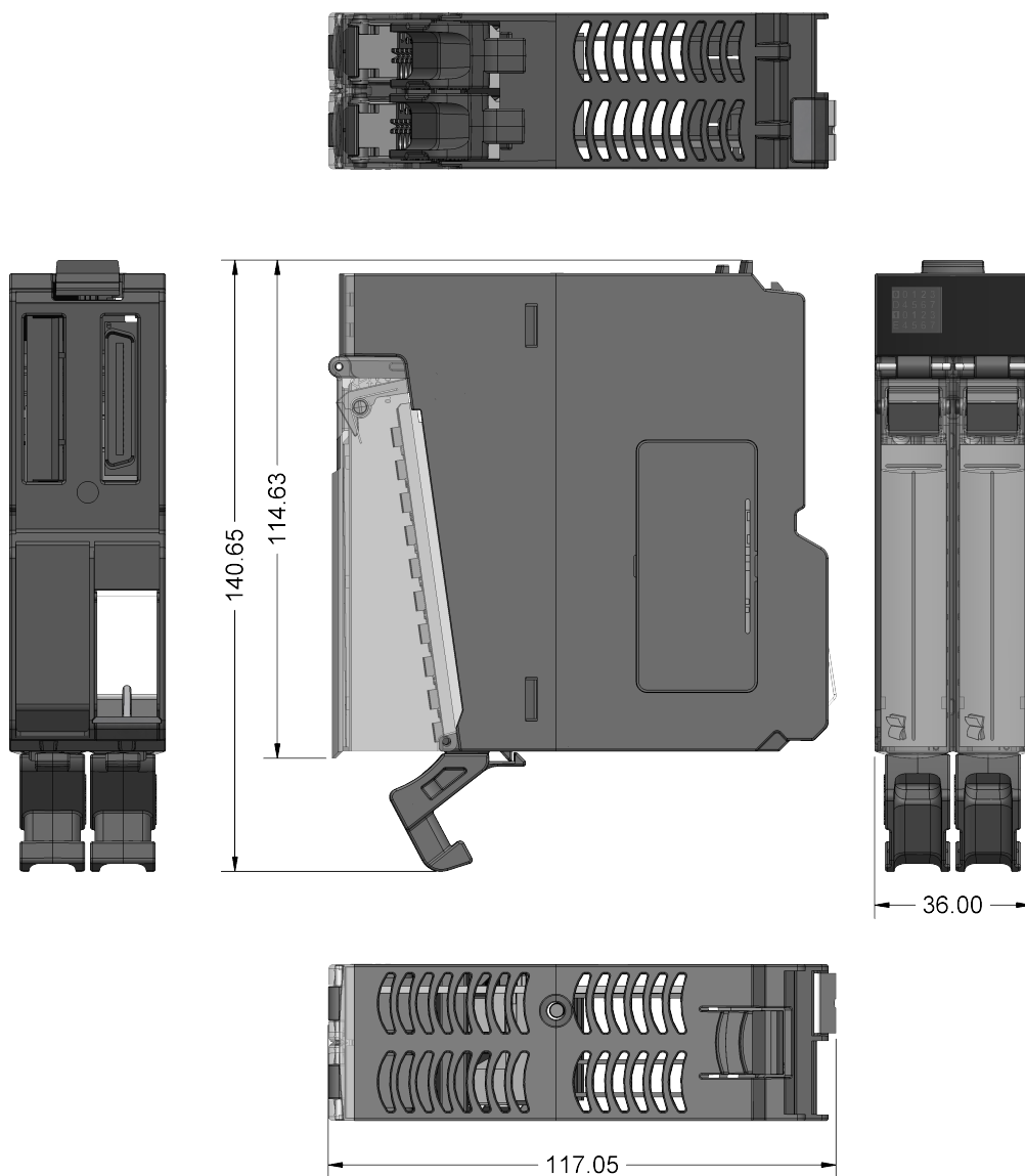
Figura 1: Dimensões Físicas
