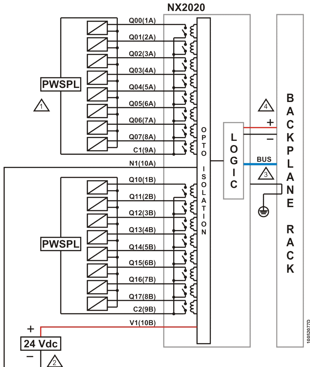
Figura 3: Diagrama Elétrico
