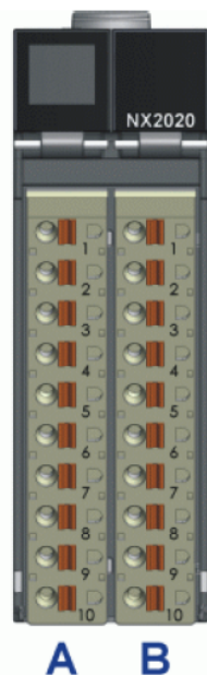
Figura 4: Pinagem do Conector
