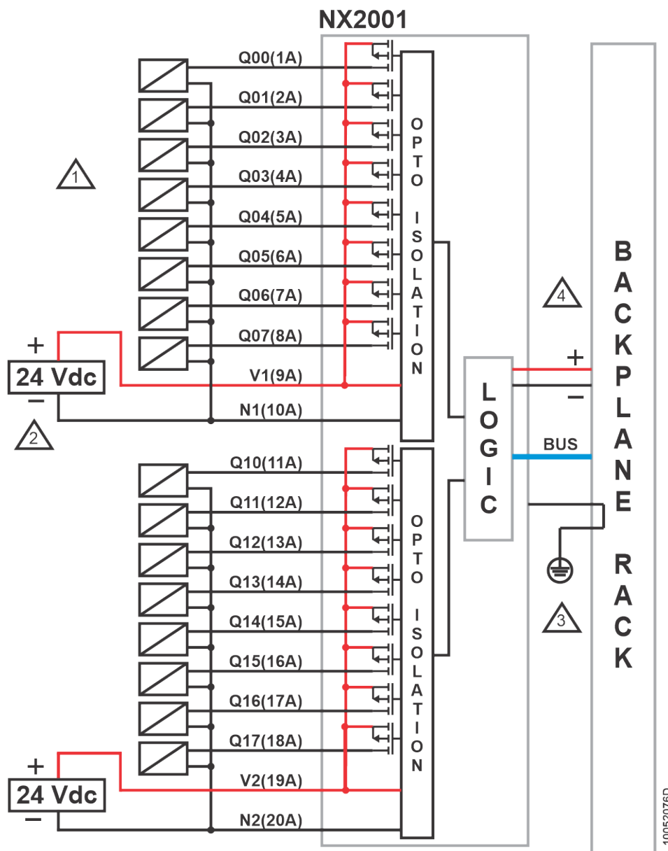
Figura 3: Diagrama Elétrico
