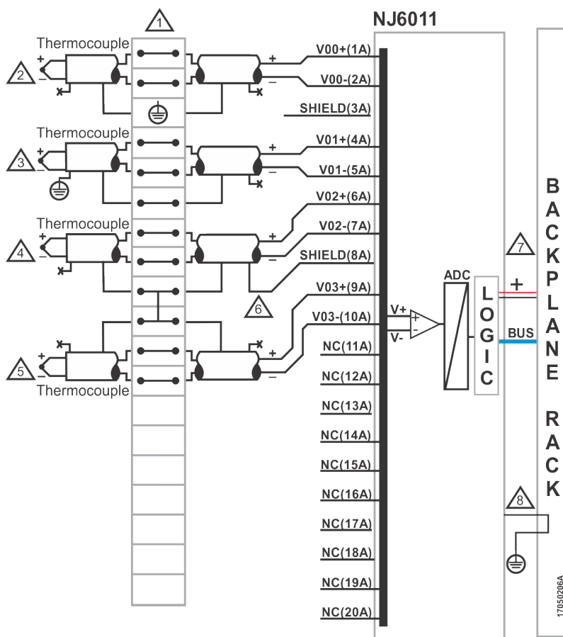
Figura 3: Diagrama Elétrico
