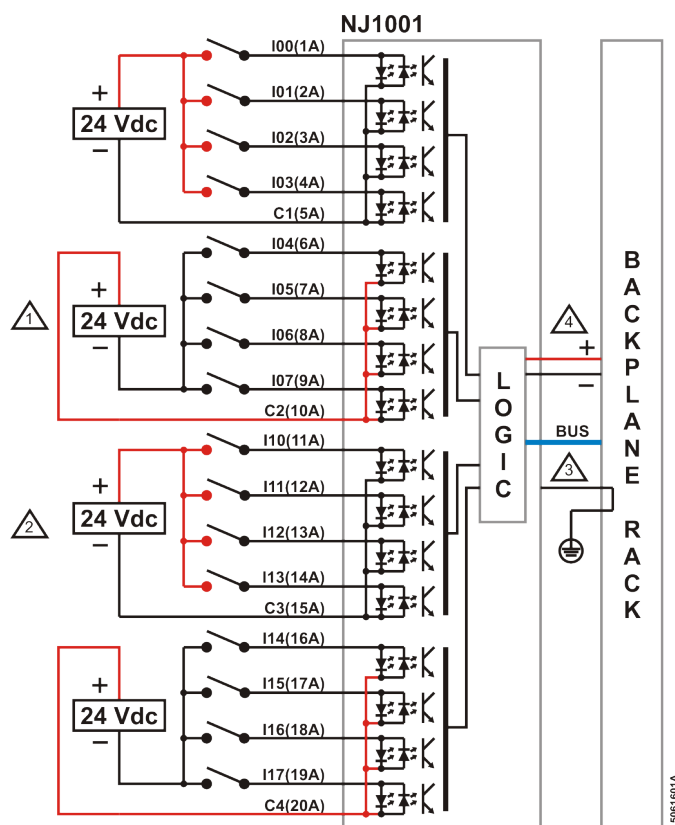
Figura 3: Diagrama Elétrico
